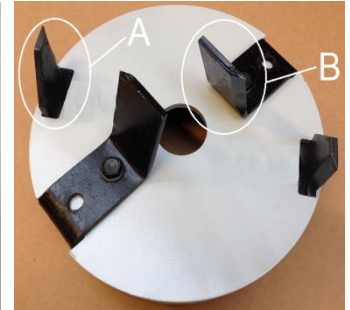
Vierer-Messerscheibe
